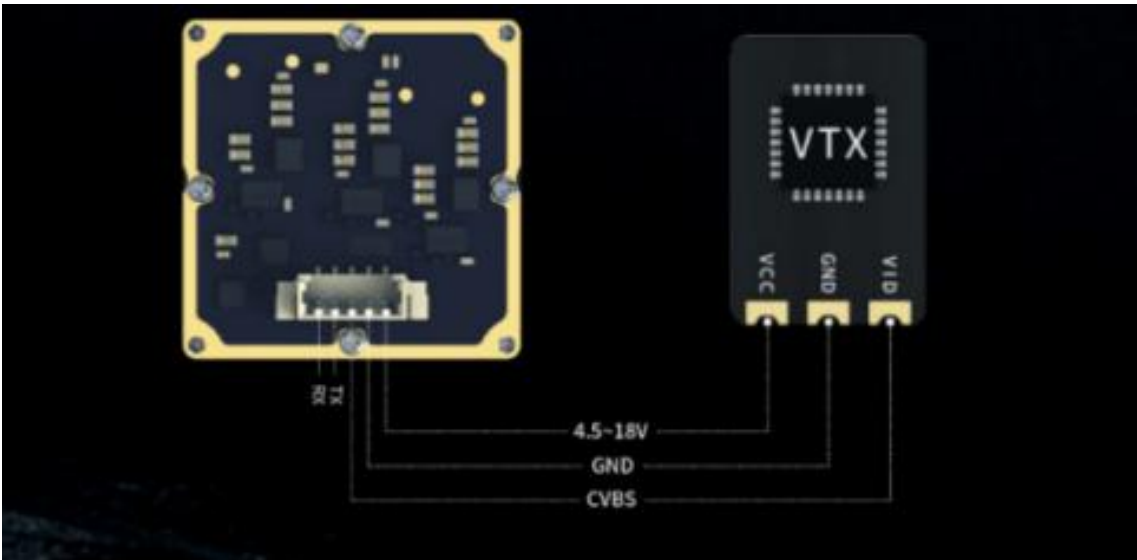
接口引脚定义图
